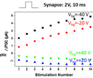
石墨烯类突触器件的结构和测试结果，通过背栅电压的调制可调制类突触器件的可塑性
