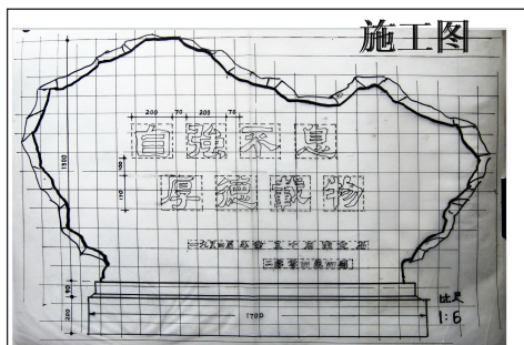
碑石的施工图
